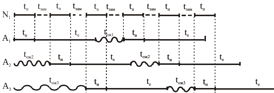
Рис. 5.2. Пример графика согласованной работы погрузчика и транспортных средств на перевозке груза:
