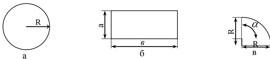
Рис. 3.1 – Расчетные схемы по формам площади пожара а – круг; б – прямоугольник; в – сектор
