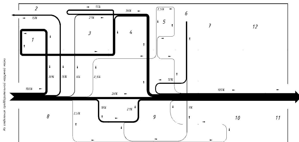
Рисунок 4.4 - Вариант прямоточной схемы грузопотоков предприятия технического сервиса:
