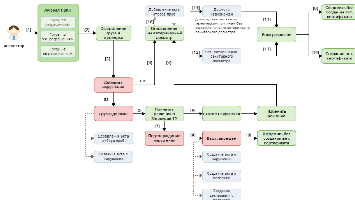
Рисунок – Схема работы в подсистеме Меркурий Подсистема Склада временного хранения «Меркурий.CBX» при импорте продукции
