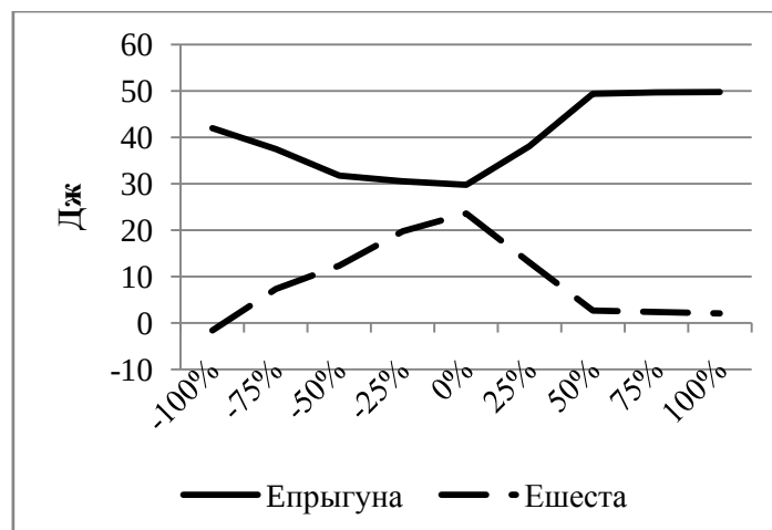
Рисунок – Механическая энергия прыгунов и деформации шеста
